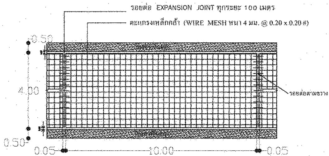
รูปแปลนผิวจราจรคอนกรีตเสริมเหล็ก
